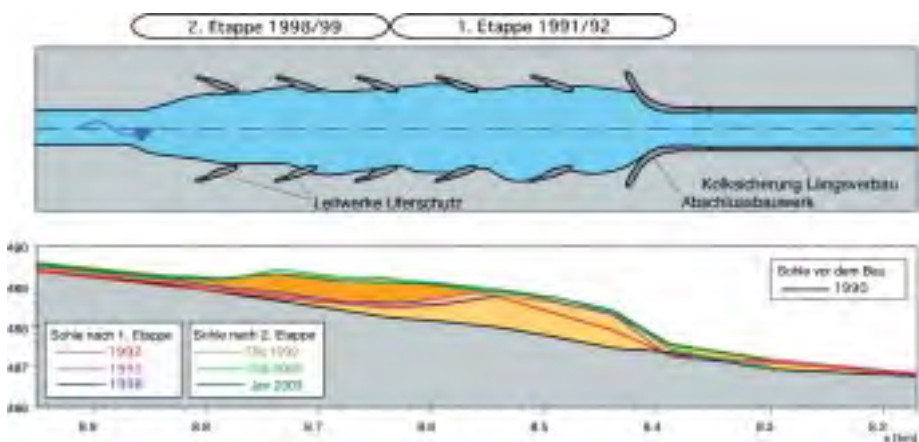
Bild 10. Situation und Längensprofil der Aufweitung «Birne Emme».
