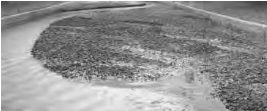
Bild 11. Verzweigtes Gerinne im hydraulischen Labor: Ausgeprägtes Verzweigungsmuster in einem Gerinne mit Ablagerungstendenz (oben) und eingetieftes Einzelgerinne bei anhaltender Erosionstendenz (unten) (Foto: VAW-ETHZ).
